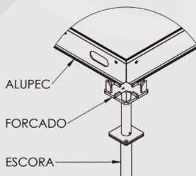
DETALHE A
